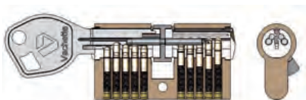
■ Cylindres profilés doubles - Réf. 7101 V5CODE - Réf. 7100 V5CODE
