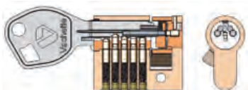
■ Cylindres profilés simples - Réf. 5101 V5CODE - Réf. 5100 V5CODE
