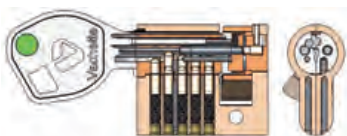
■ Cylindres profilés simples - Réf. 5101 V5CODE N1 - Réf. 5100 V5CODE N1
